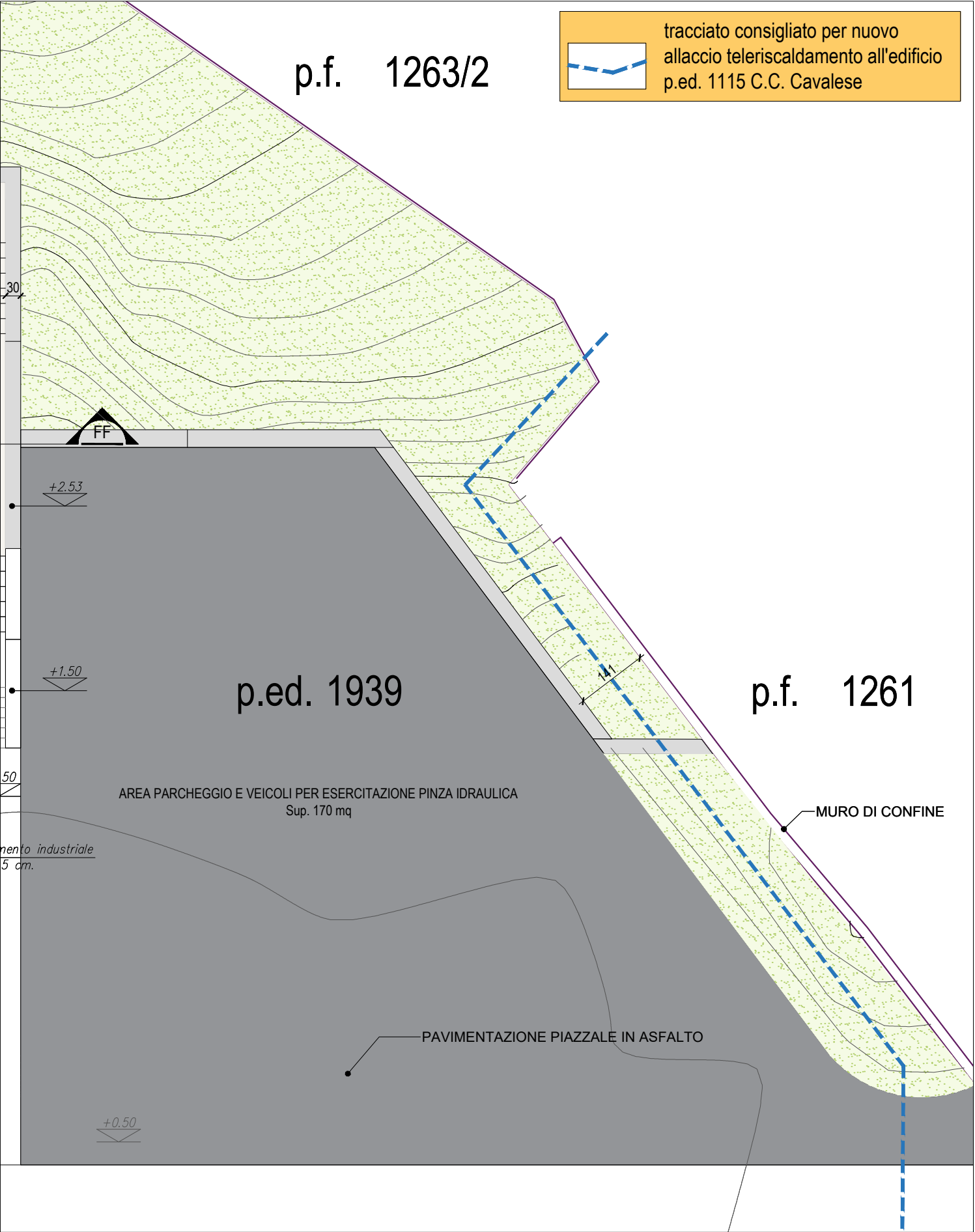
01 PLANIMETRIA PARCHEGGIO - STATO DI PROGETTO 1:100
